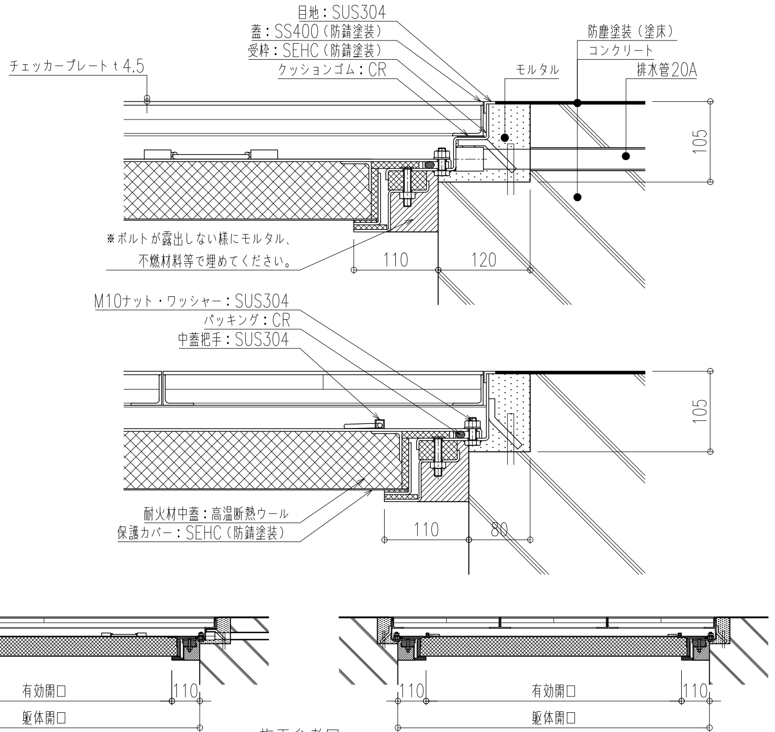
施工参考図
